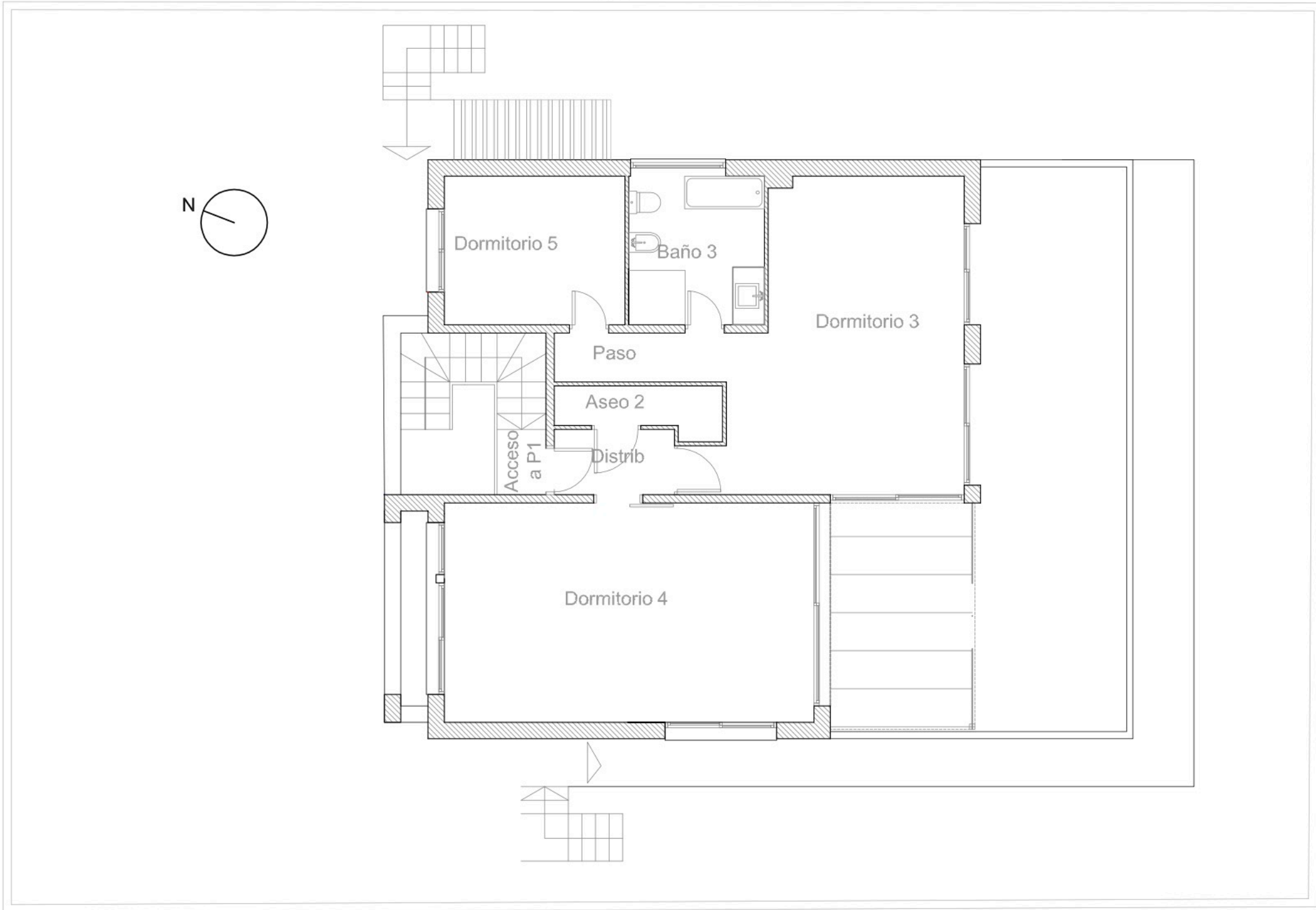
PLANTA PRIMERA
