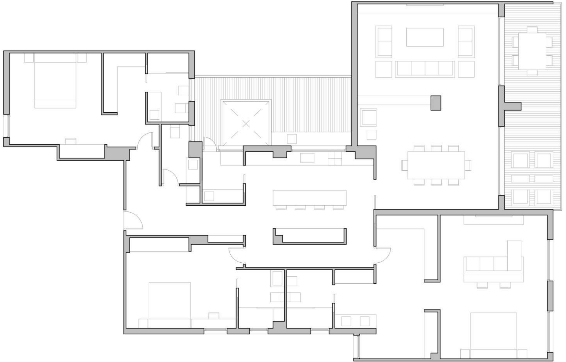
PROPUESTA REFORMA
