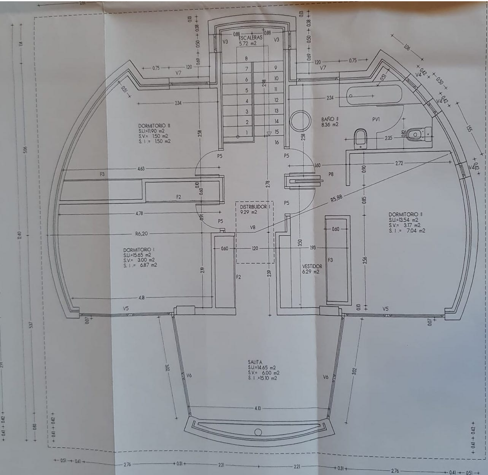
PLANTA PRIMERA
