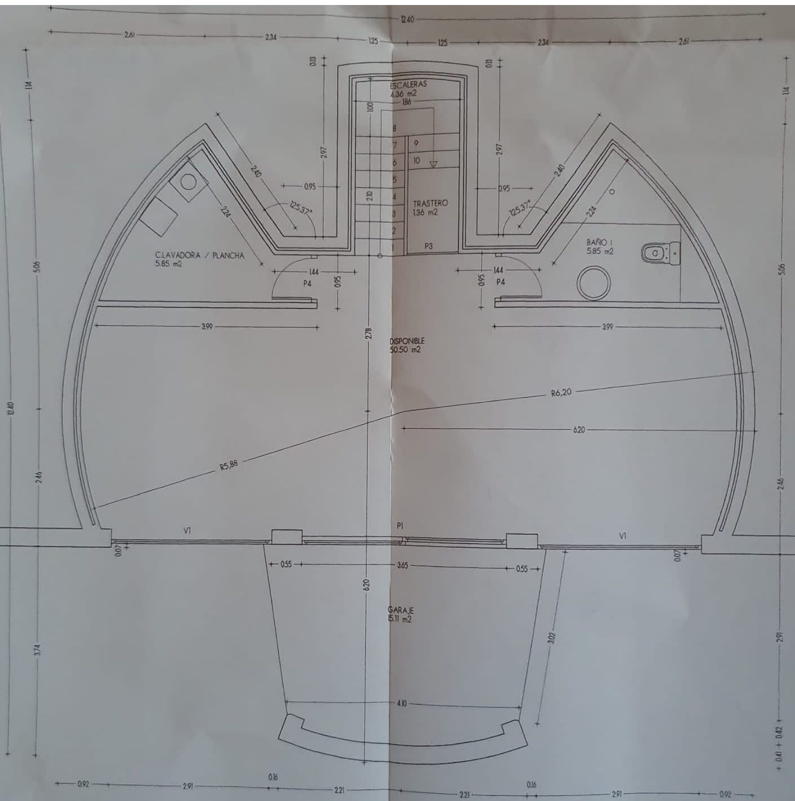
PLANTA SEMISOTANO
