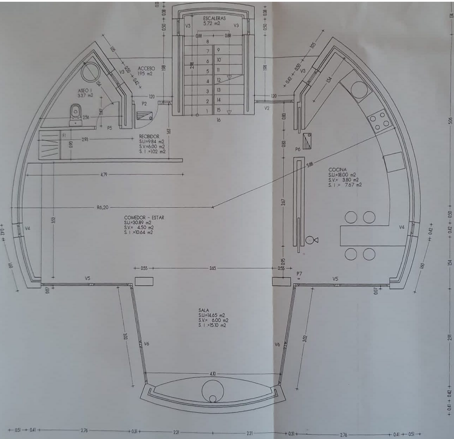
PLANTA BAJA
