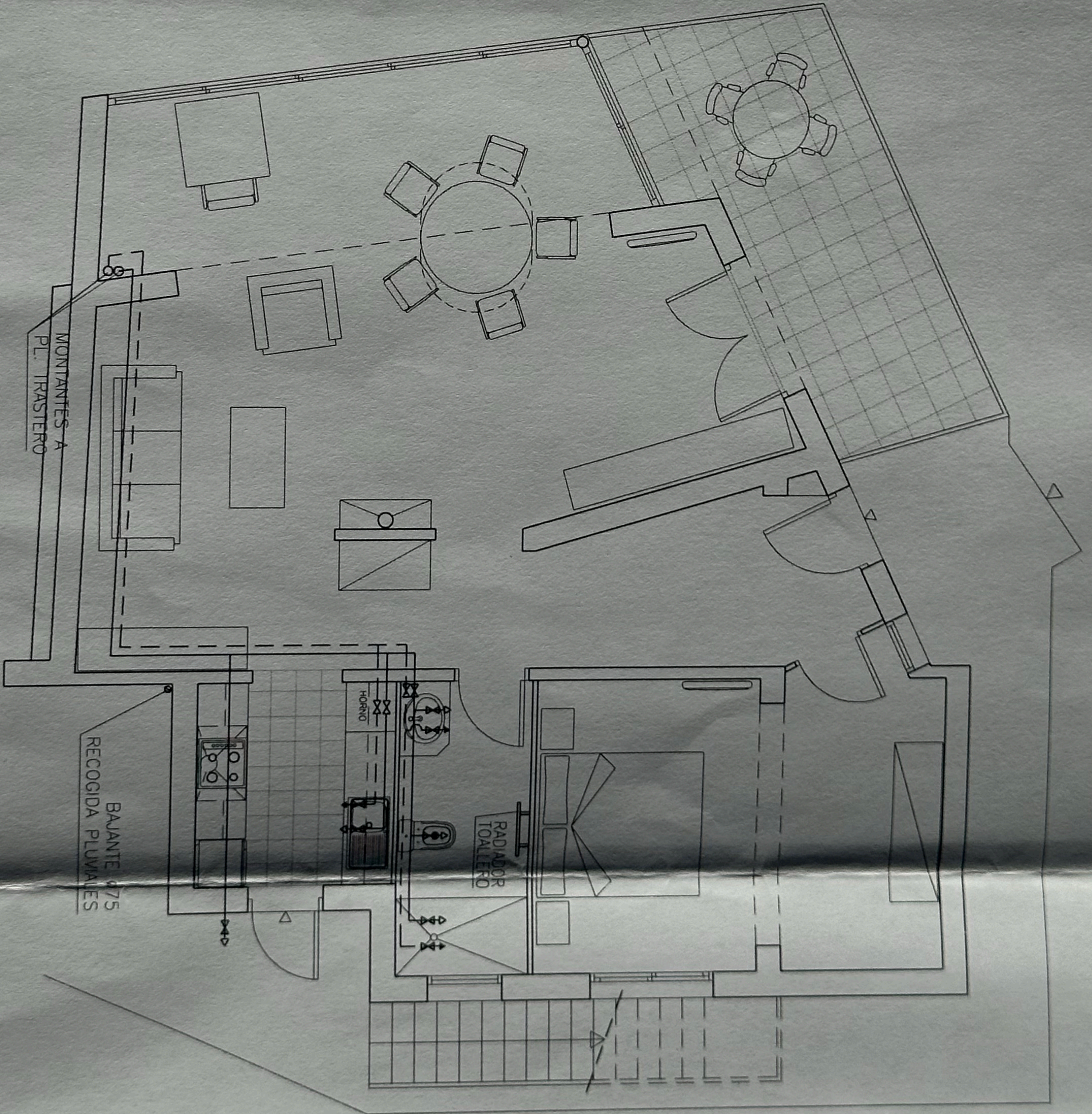
PLANTA BAJA E:1/50
